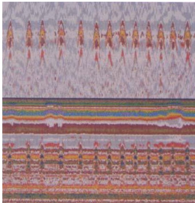
รูปที่ 4 ภาพขยายสัญญาณจากวิธีเรดาร์ (Ground-penetrating radar) (ที่มาจาก Gary Crawford, FHWA)
